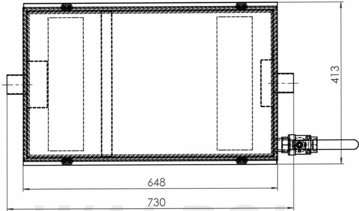
Draufsicht M 1:6
