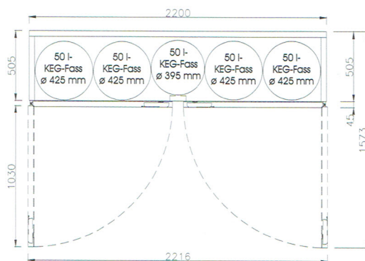
FK 5 / 2-türig
