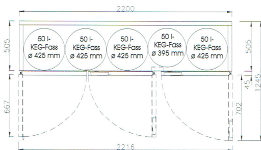
FK 5 / 3-türig
