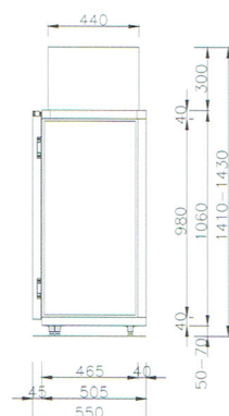
Schnitt Fasskühler einreihig
