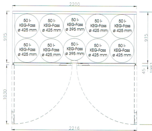
Schnitt Fasskühler zweireihig
