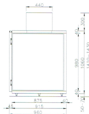
Schnitt Fasskühler zweireihig
